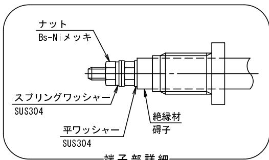
端子部詳細
